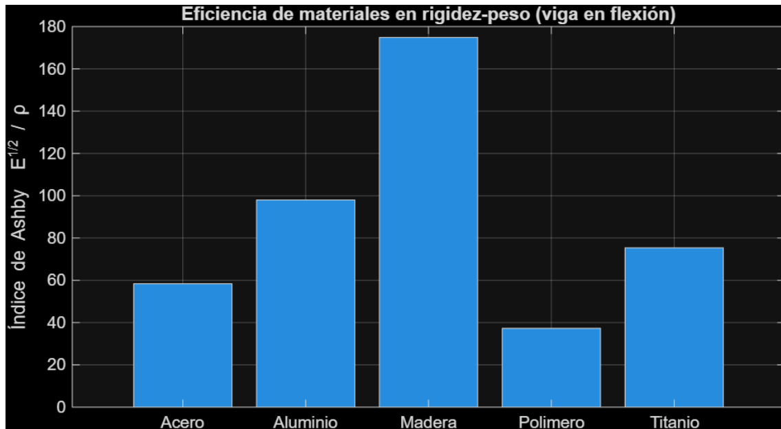
Figura 2: Eficiencia Rigidez / Peso de materiales.
